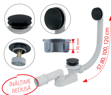
A507BLACK Ventil cadă CLICK/CLACK cu sifon, negru-mat
